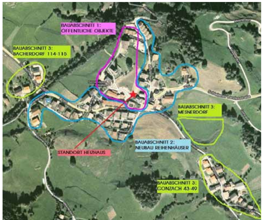
Aus der Projektmappe der Firma ProPlan: Die Einteilung der einzelnen Bauabschnitte der vorgestellten Nahwärmeversorgungsanlage in Schlaiten.
